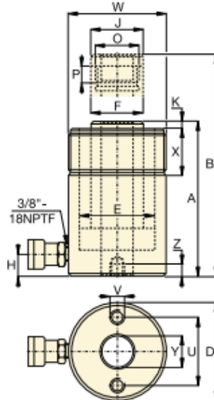
Modellerna RCH-202 - RCH-1003
