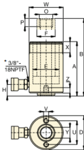
Modellerna RCH-120 - RCH-123 * 1/4" NPTF för RCH-120
